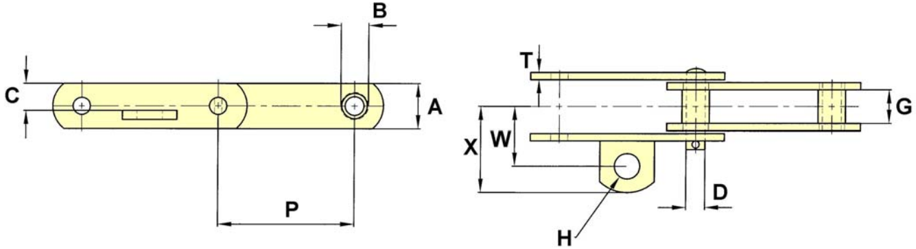
Welded Lug
